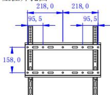
壁挂开孔图
