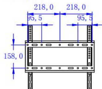
壁挂开孔图
