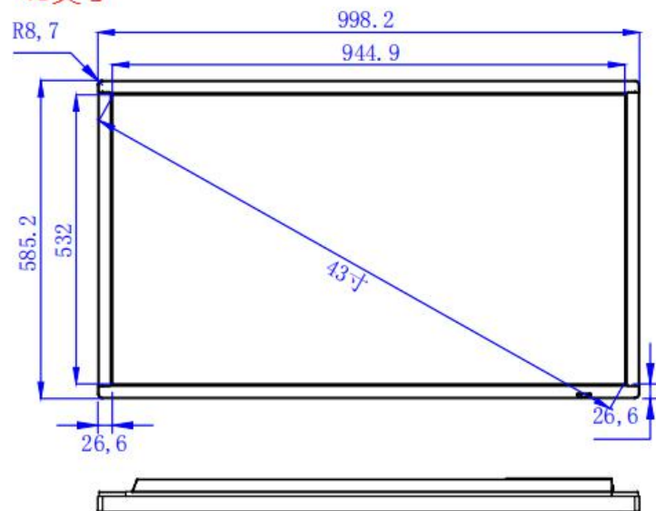
壁挂开孔图
