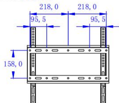
壁挂开孔图
